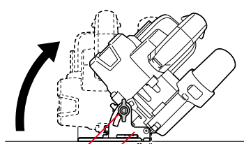
夾緊螺絲 斜切刻度板
